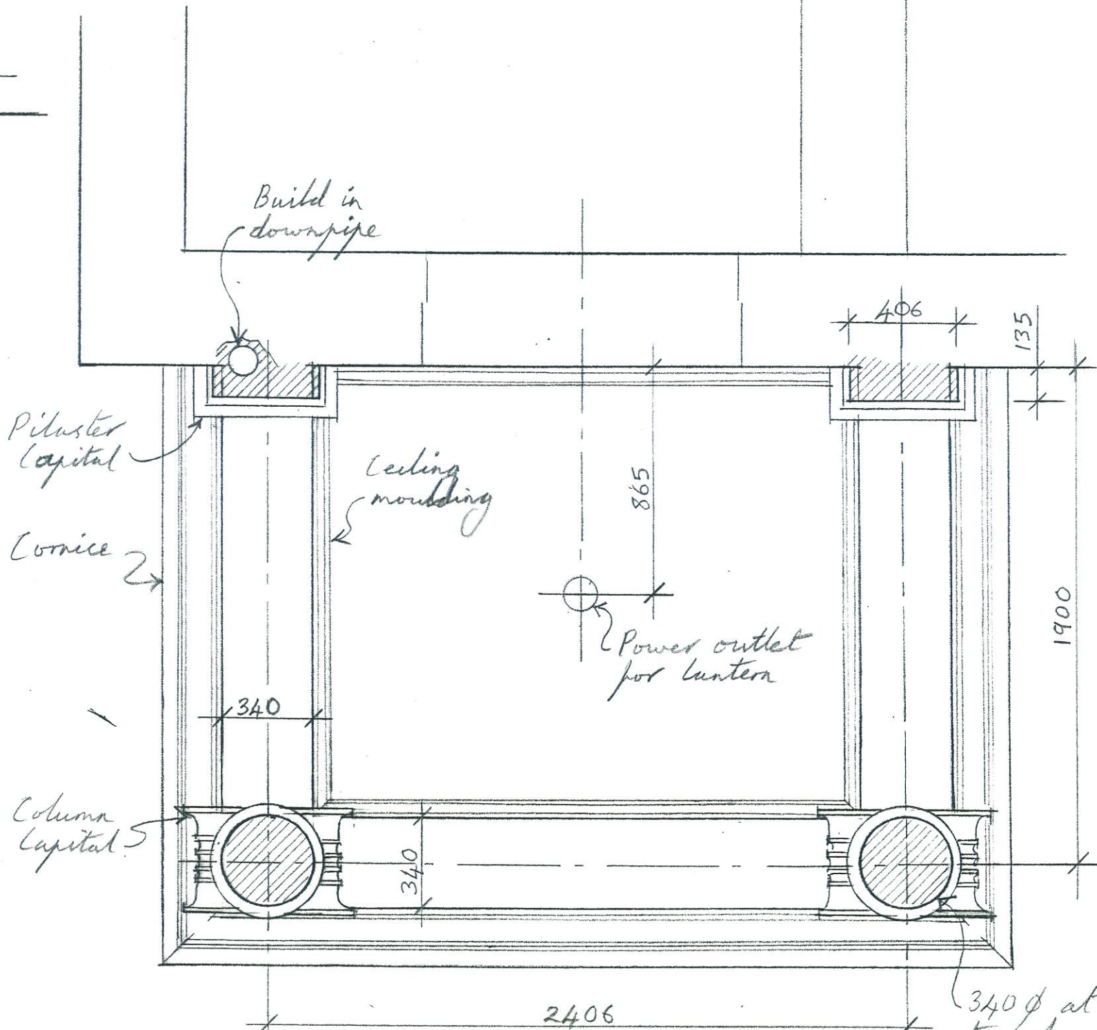
Column Capital 1:5
